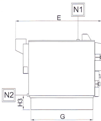
PROSPETTO LATERALE Sx lateral view side Sx
