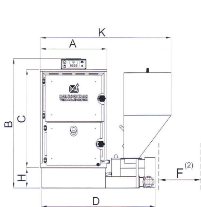
PROSPETTO ANTERIORE frontal view
